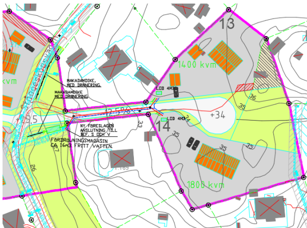
Figur 14. Föreslagna VA- och dagvattenlösningar för delområde C. (Bild: AFRY)
