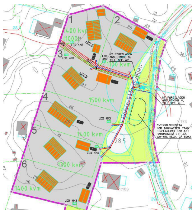
Figur 12. Föreslagna VA- och dagvattenlösningar för delområde A. (Bild: AFRY)
